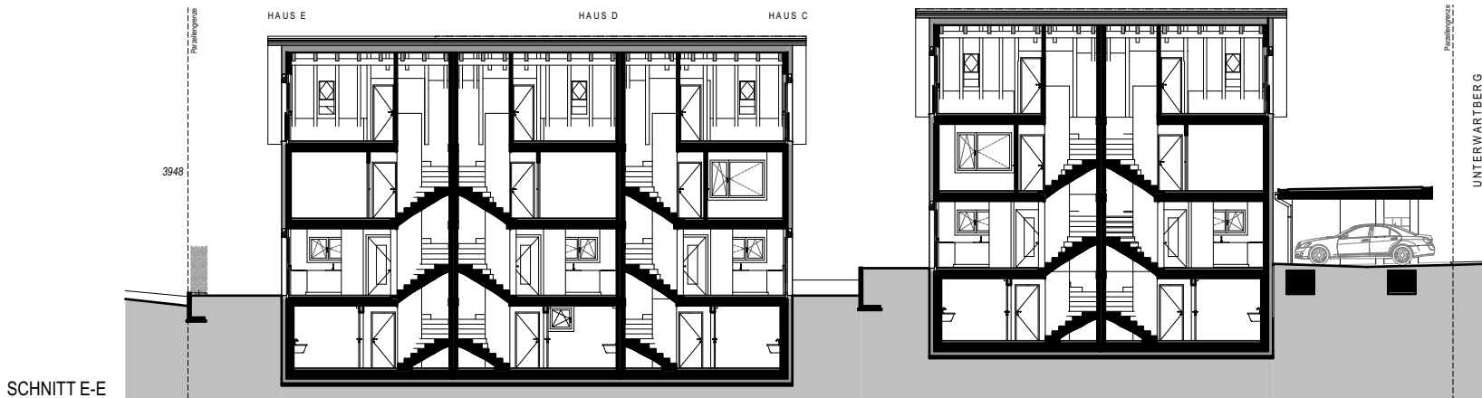
SCHNITT E-E
